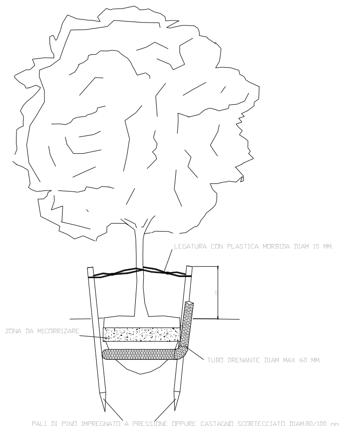
Fig.1) Schema di impianto e posizionamento del tubo per l'irrigazione manuale
